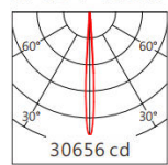
XP-E2 7° 2700K
