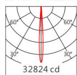
XP-E2 7° 3000K
